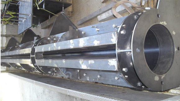
溶銑予備処理用インジェクションランス施工枠
